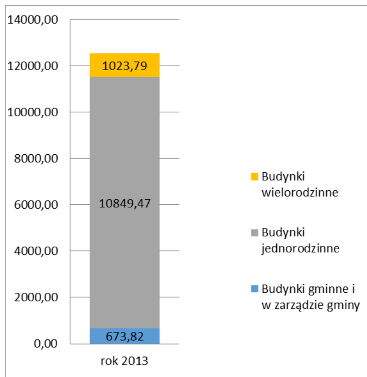
Wykres 8. Wielkość emisji CO 2 związana ze spalaniem paliw do celów energetycznych [MgCO 2 /rok]
