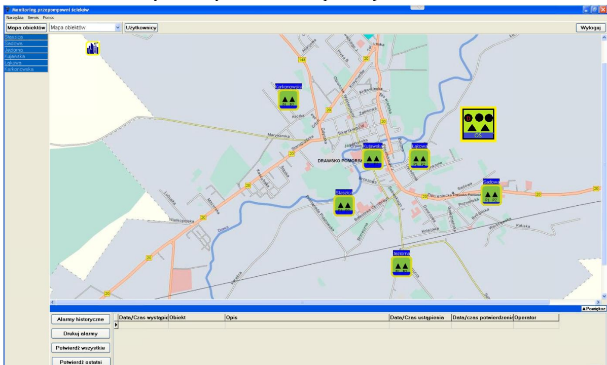
Główne okno synoptyczne wizualizujące monitorowane obiekty.
